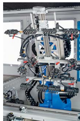
Automatisch verstellbarer Saugrahmen Automatically adjustable gripper
